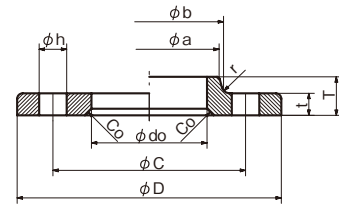
SOP-LJ
