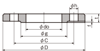
SOP-RF
