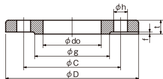
SOP-RF
