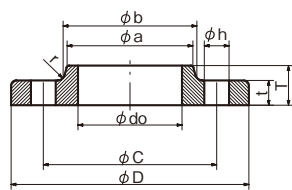
SOH-FF
