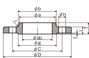
SOH-RF
