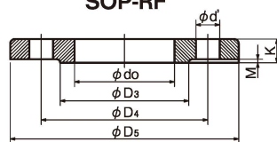
SOP-RF
