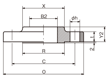
SO-RF
