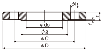
SOP-RF
