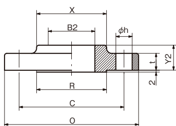
SO-RF
