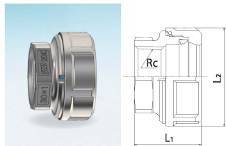
NJXFA めすアダプタ
