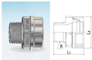
NJXMA おすアダプタ
