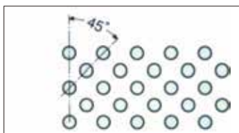
角千鳥(45°)
