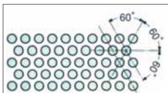
千鳥(60°)
